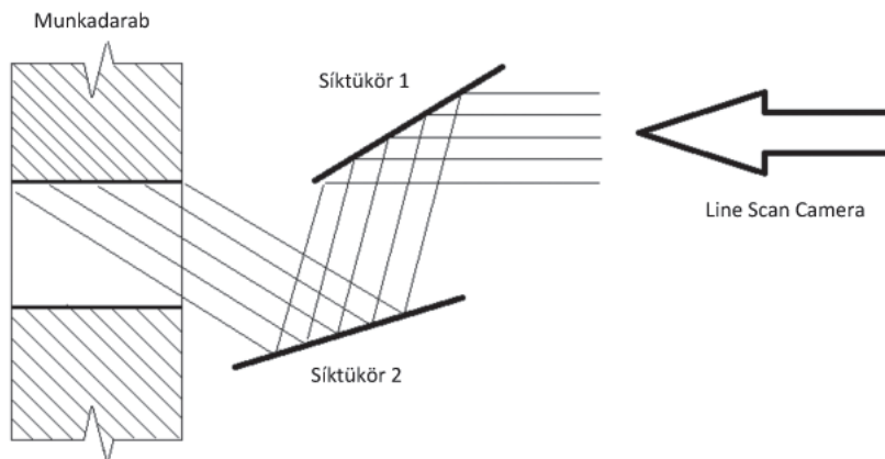
15. ábra. Tükörrendszer felépítésének a vázlata
