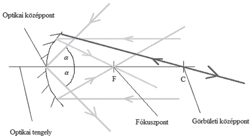
9. ábra. Homorú tükörről történő visszaverődés
