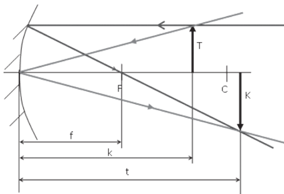
11. ábra. Homorú tükör képképzés fókusz és a görbületi középpont között lévő tárgynál
