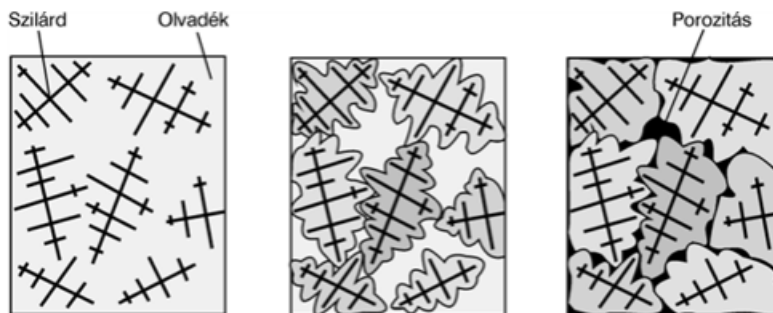
1. ábra. Porozitás-kialakulás [2]
