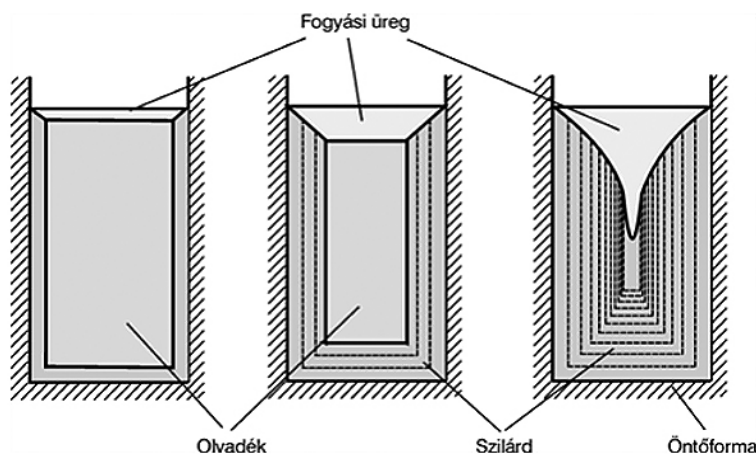
2. ábra. Lunker-kialakulás [2]
