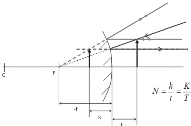
14. ábra. Domború tükör képalkotása
