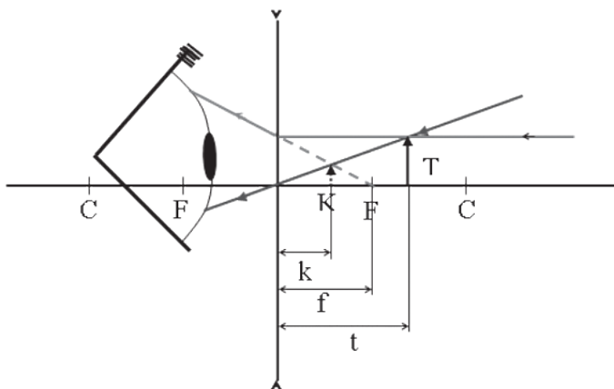
5. ábra. Szórólencsés képalkotás
