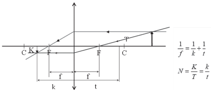
4. ábra. Gyűjtőlencsés képalkotás
