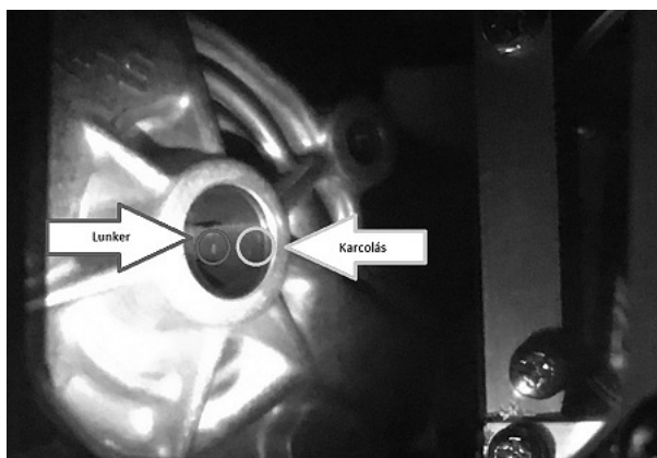
18. ábra. 50 mm tükör segítségével történő vizsgálat
