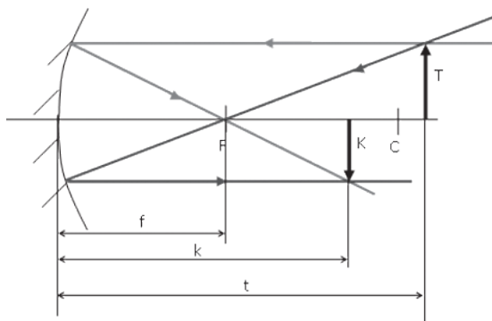
10. ábra. Homorútükör-képképzés 2-szeres fókusz távolságon kívüli tárgynál
