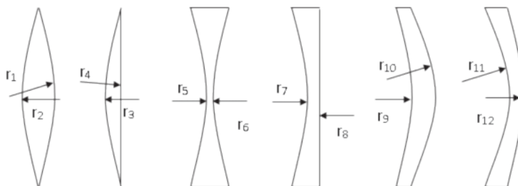
3. ábra. Lencse típusok
