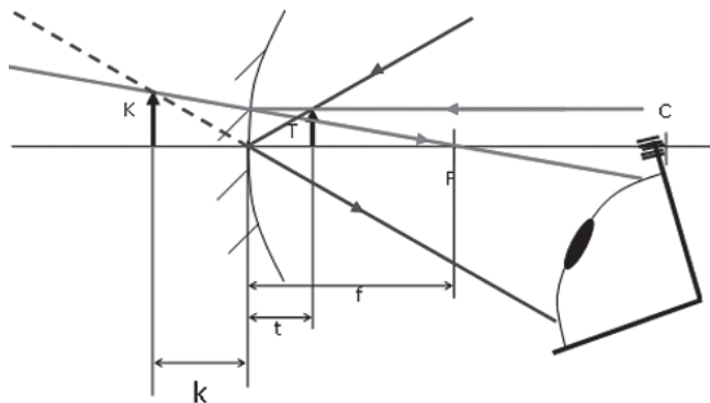
12. ábra. Homorú tükör képalkotása fókuszpont és a tükör között lévő tárgynál
