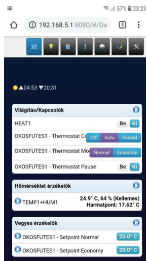
16. ábra. Domoticz kezelőfelülete mobil eszközön.
