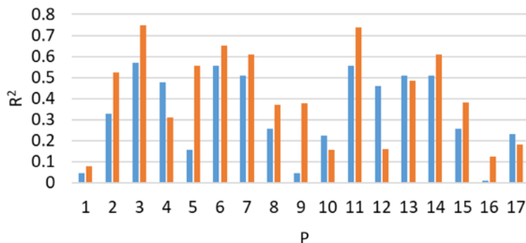
6. ábra. Korrelációs vizsgálat eredményei az egyes prediktorok és a PM_{10} -koncentráció értékei között Veszprémben (kék) és Miskolcon (narancs).
