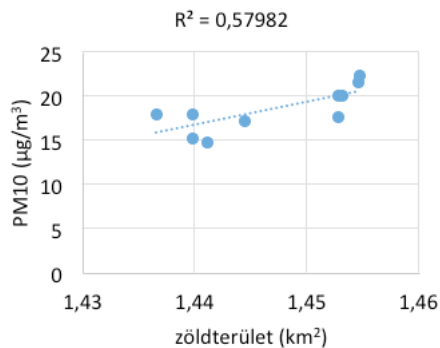
5. ábra. Az egyes városi tényezők és a PM_{10} -koncentráció korrelációs vizsgálatának eredménye (bal oldal), valamint külön ábrázolva a zöldterületek és PM_{10} -koncentráció közötti lineáris kapcsolat vizsgálata (jobb oldal).
