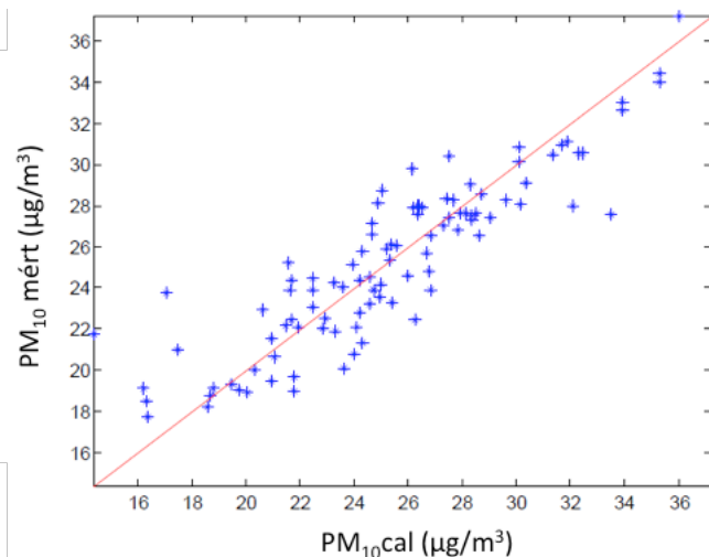
8. ábra. Számított és valós PM_{10} -koncentráció (M12).
